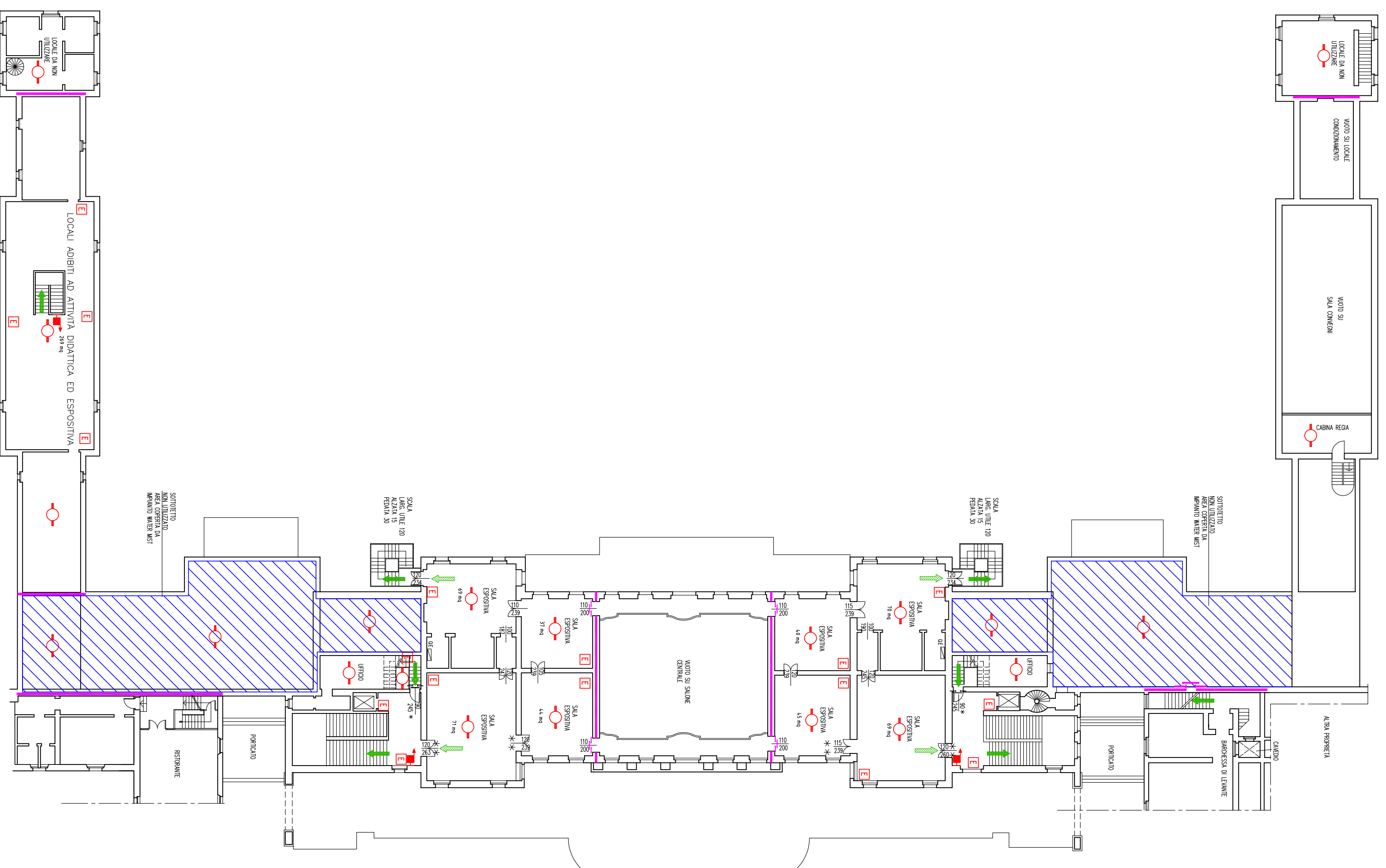
CORPO CENTRALE E AI POSTICHE PIANTA PIANO PRIMO
